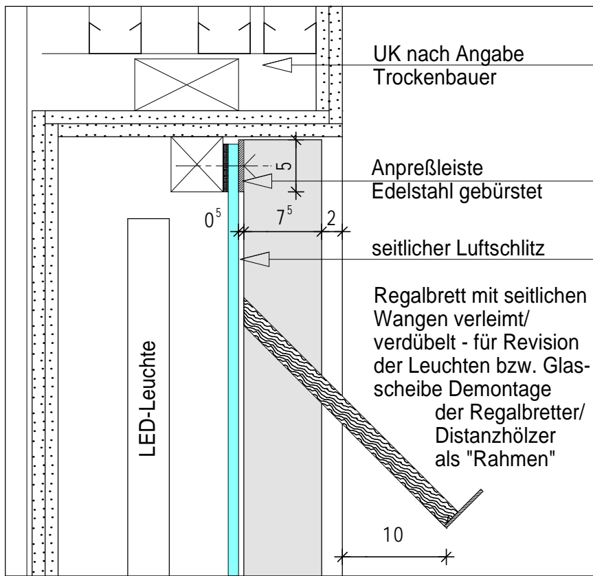
Vitrine 1 - Vertikalschnitt 1-1 M 1:5
