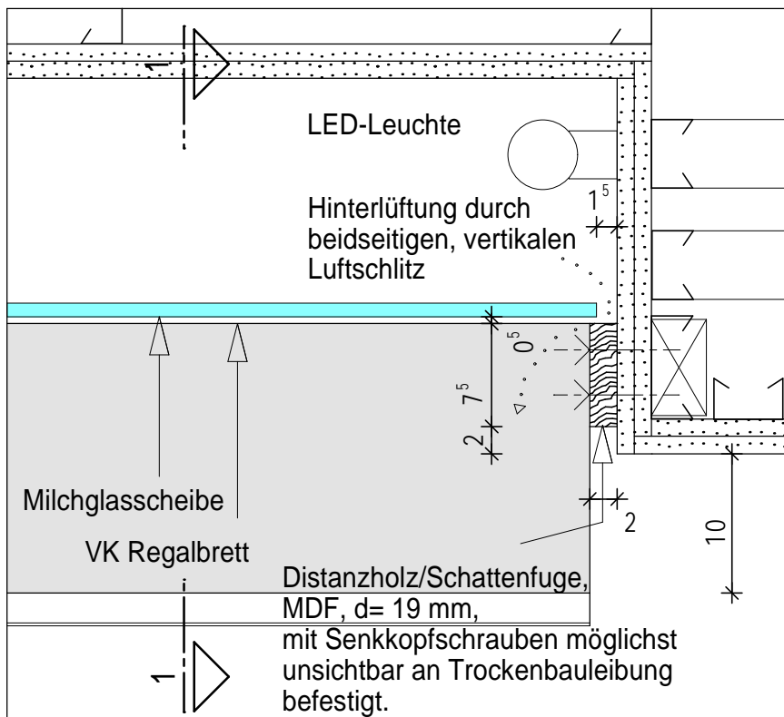
Vitrine 1 - Horizontalschnitt 2-2 M 1:5
