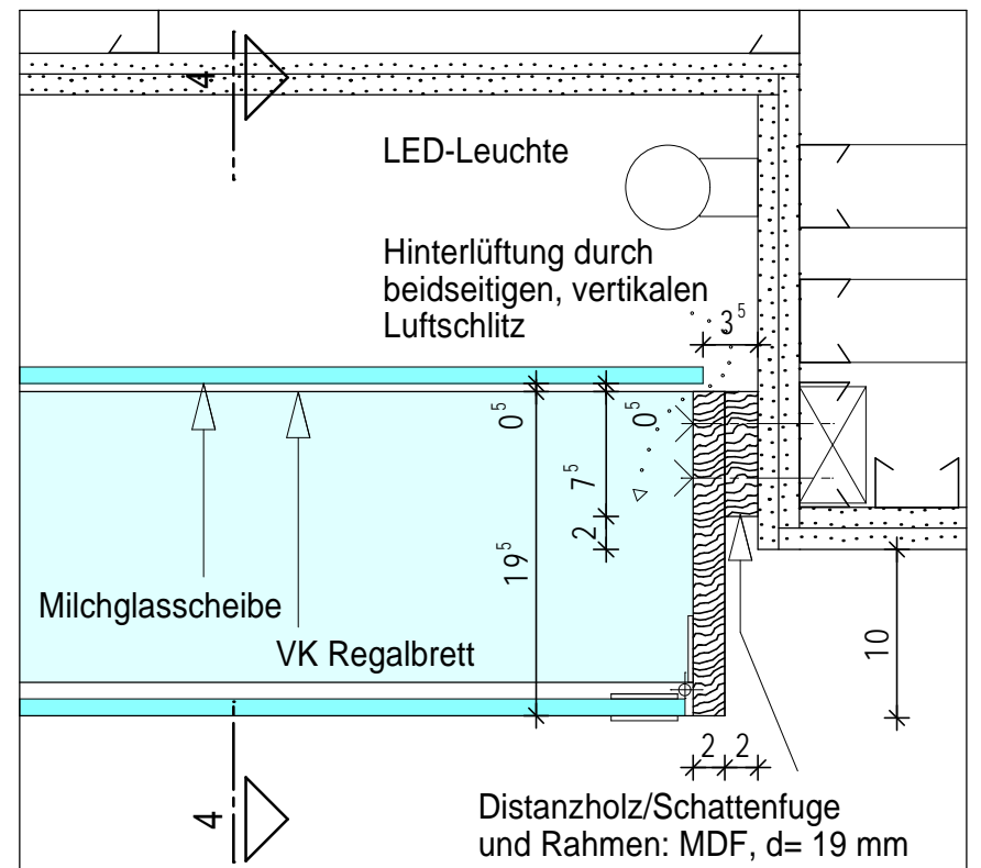
Vitrine 2 - Horizontalschnitt 4-4 M 1:5
