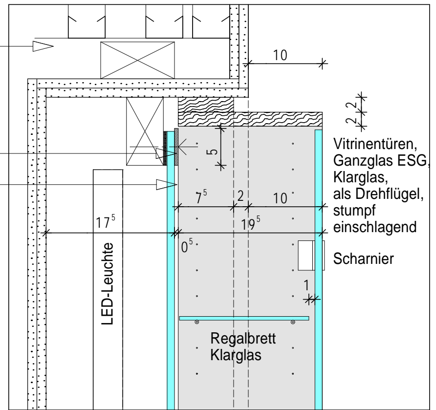
Vitrine 2 - Vertikalschnitt 3-3 M 1:5
