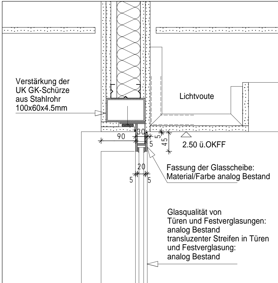
Anschluß Glaswand/Glastür an GK-Schürze Vertikalschnitt M 1:5
