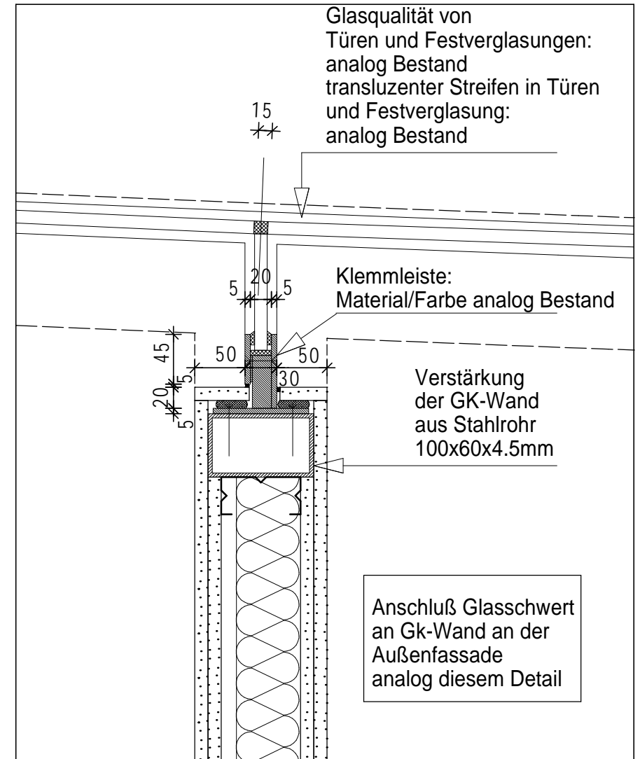
Anschluß GK-Wand an Glaswand Horizontalschnitt M 1:5
